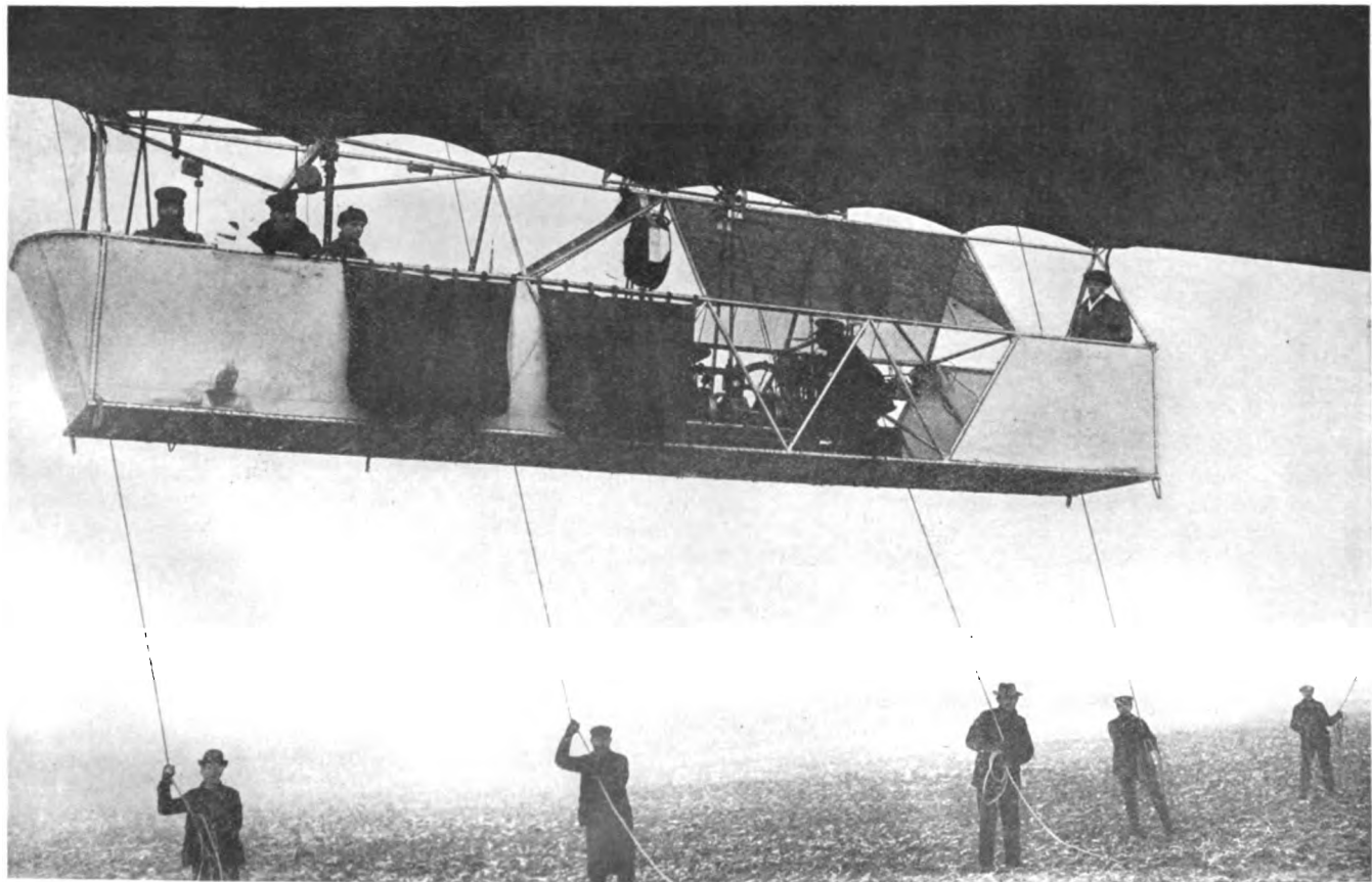
THE CENTRAL CAR OF THE S. S. J.
