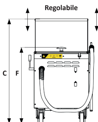
Vista frontale
