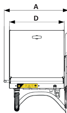
Draufsicht
