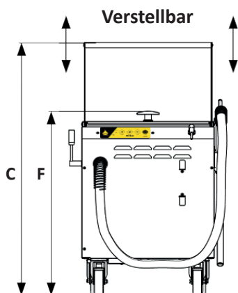
Vorderansicht
