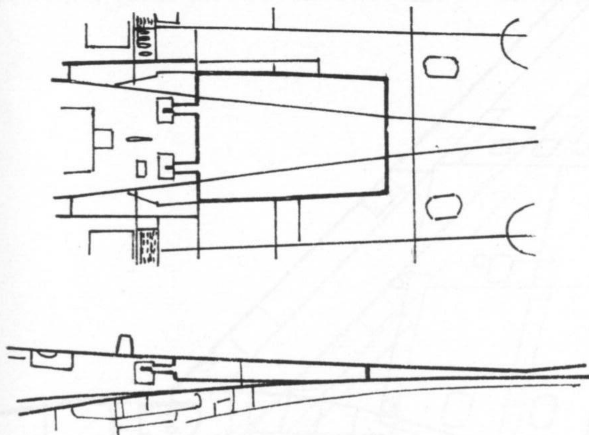
Particolare dell'aerofreno più piccolo dei primi esemplari
